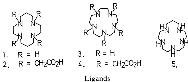
Fig. 1. Ligands: 1. [14]aneN 4 (Cyclam); 2. [14]aneN 4 -tetraacetic acid; 3. [15]aneN 5 ; 4. [15]aneN 5 -pentaacetic acid; 5. [16]aneN 5 .
